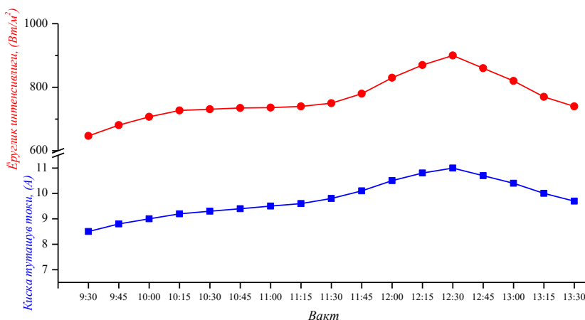
2-rasm. FES yuzasiga tushayotgan yorug'lik intensivligi va qisqa tutashuv tokining kunduzgi vaqtga bog'liqligi
