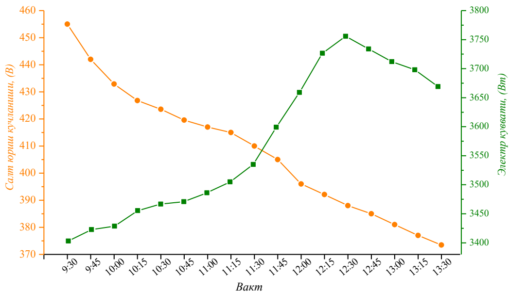
3-rasm. FES salt yurish kuchlanishi va elektr quvvatining kunduzgi vaqtga bog‘liqligi
